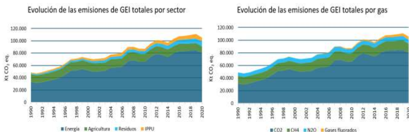
Ilustración 3: Evolución de las emisiones de GEI por sector y por gas (Elaboración propia con base en Dirección Meteorológica de Chile 2022)
