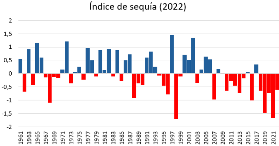
Ilustración 6: Índice de sequía a nivel nacional (Elaboración propia con base en Dirección Meteorológica de Chile 2022))
