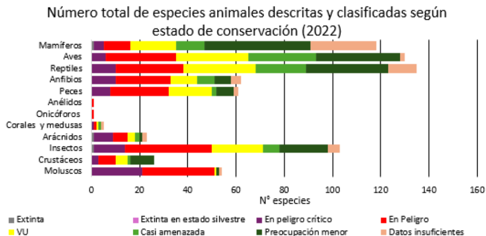
Ilustración 7: Número total de especies de animales según estado de conservación (Elaboración propia)
