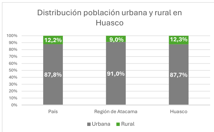
Ilustración 32: Población urbana y rural de Huasco (Elaboración propia en base al Censo 2017)
