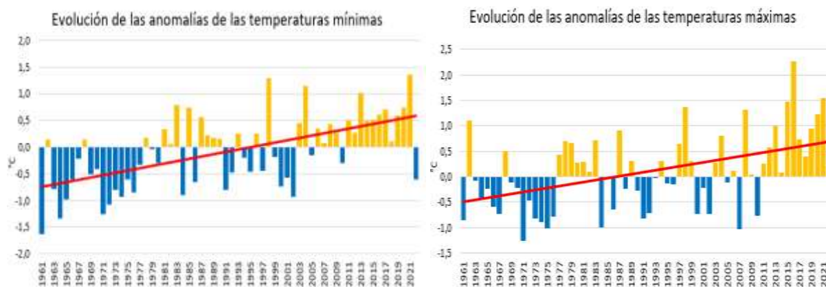
Ilustración 2: Evolución de las anomalías de las temperaturas mínimas y máximas (Elaboración propia con base en Dirección Meteorológica de Chile 2022)
