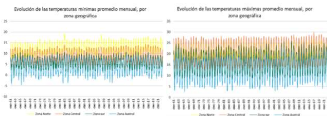
Ilustración 1: Evolución de las temperaturas mínimas y máximas promedio por zona geográfica (Elaboración propia con base en Dirección Meteorológica de Chile, 2022)
