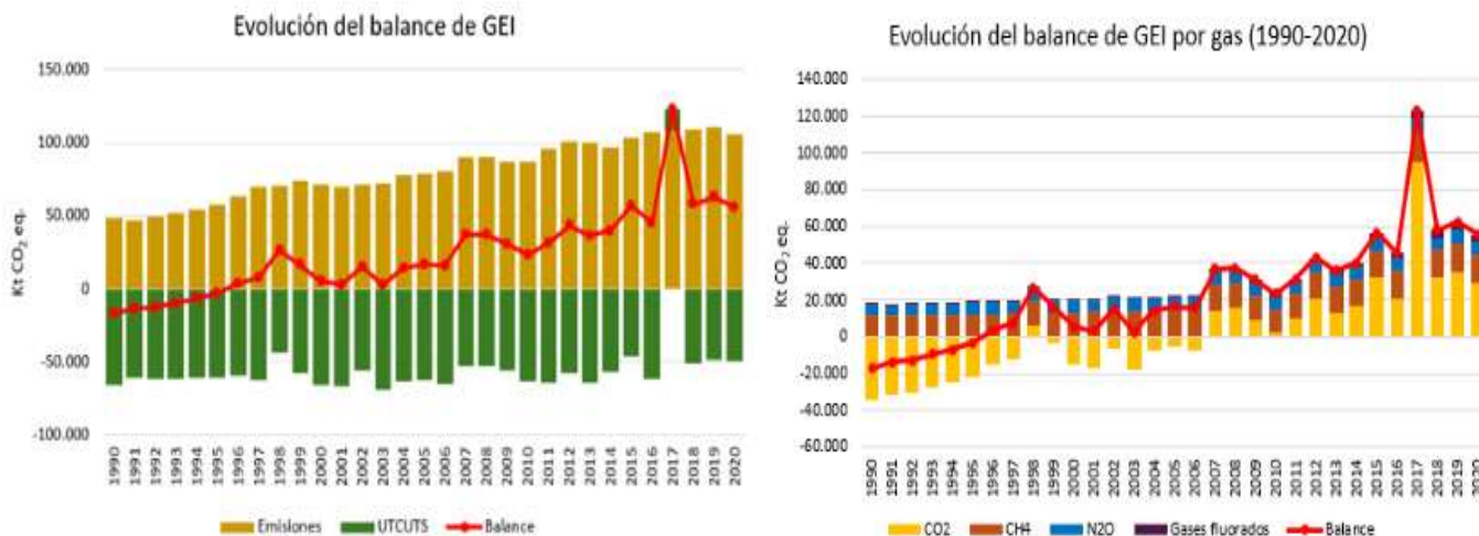
Ilustración 4: Evolución del balance de GEI (Elaboración propia con base en Dirección Meteorológica de Chile 2022)
