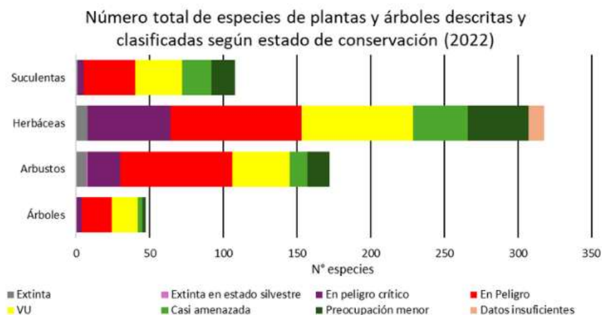
Ilustración 8: Número total de especies de plantas y árboles según estado de conservación (Elaboración propia)
