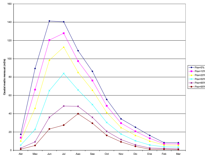
Figura 4.9: Curva de Variación Estacional Río Donguil en Gorbea
