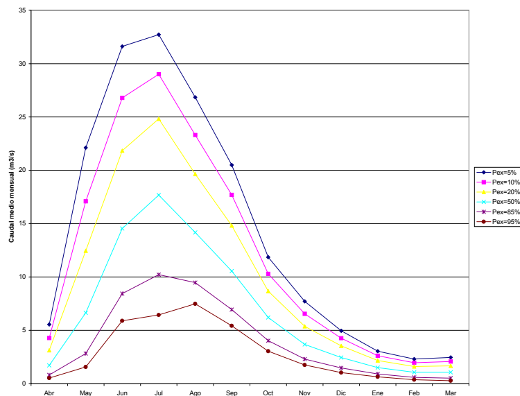
Figura 4.8: Curva de Variación Estacional Río Puyehue en Quitratue
