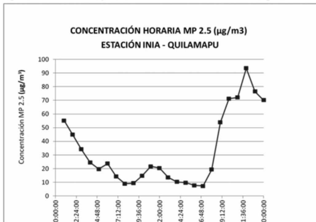
Figura N°4. Ciclo diario de MP2,5 representativo de un día de invierno en base a promedios horarios de junio de 2010 en Estación INIA - Quilmapu de Chillán
