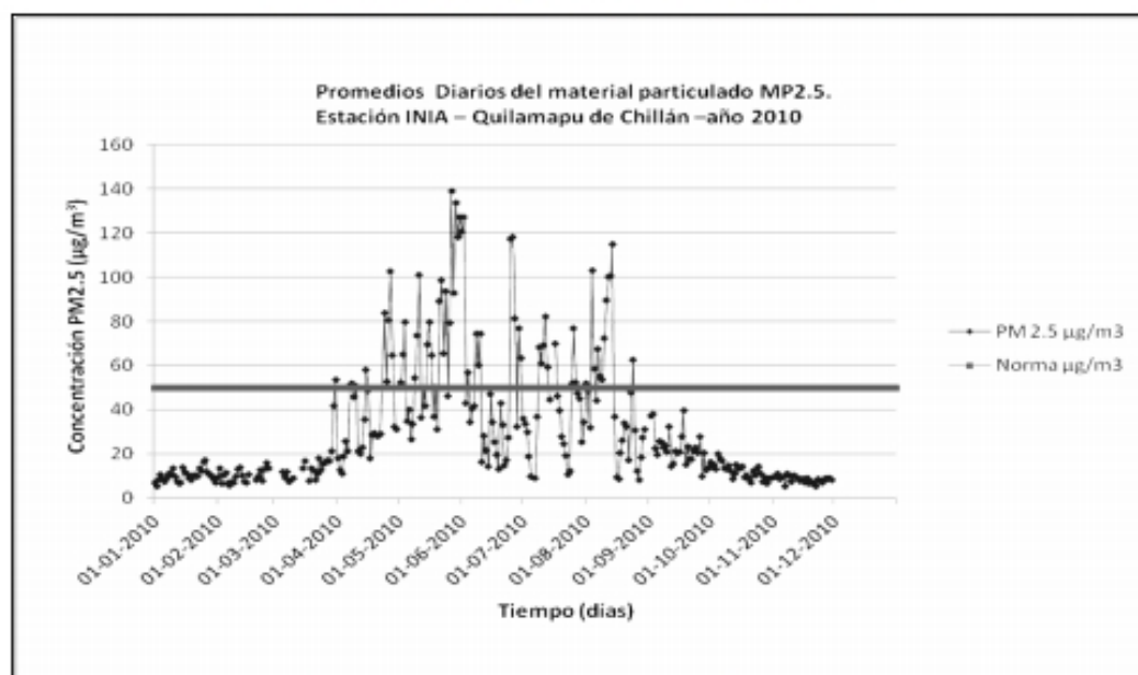
Figura N°3. Promedios diarios del Material Particulado MP2,5 Estación INIA - Quilamapu de Chillán - año 2010
