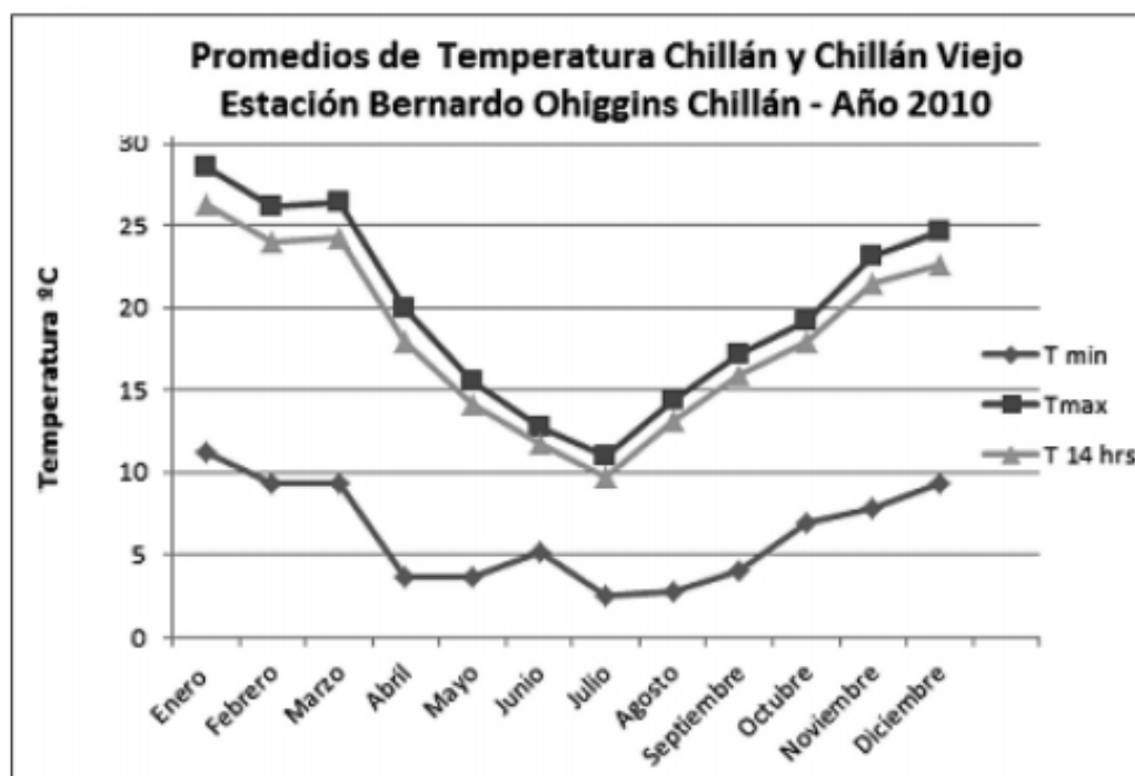
Figura N°1. Promedios mensuales de temperatura Año 2010
