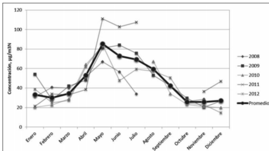
Figura N°2. Promedios mensuales del Material Particulado MP 10 , Estación INIA - Quilamapu
