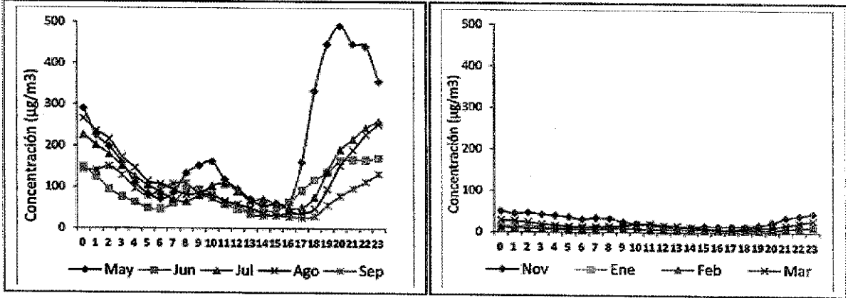
Figura 5: Ciclo de concentración diaria de MP2,5 (año 2010)
